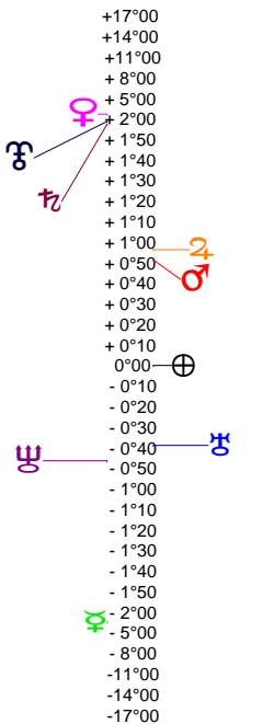
Latitudes héliocentriques
