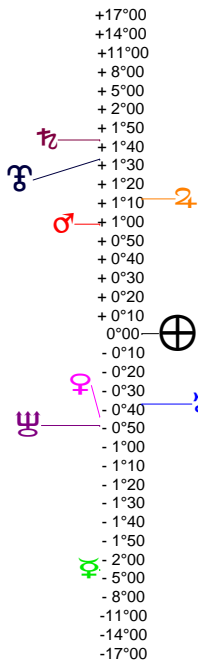
Latitudes héliocentriques
