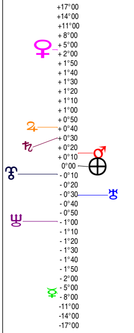
Latitudes héliocentriques
