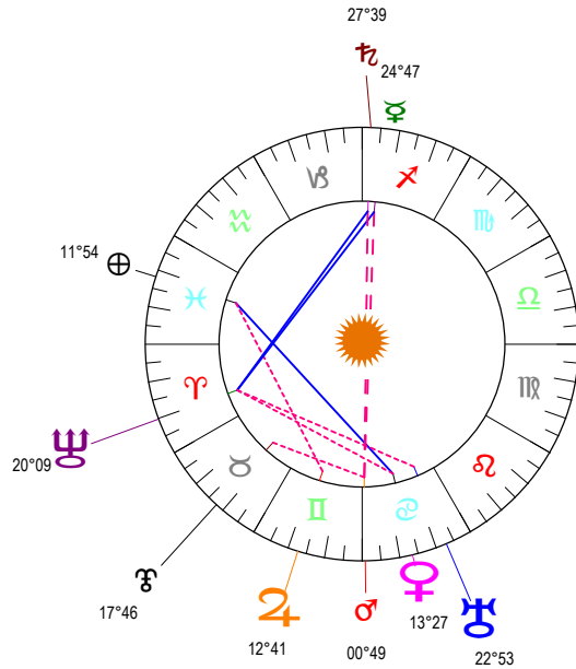
Sphère hélio-écliptique - Intégration
