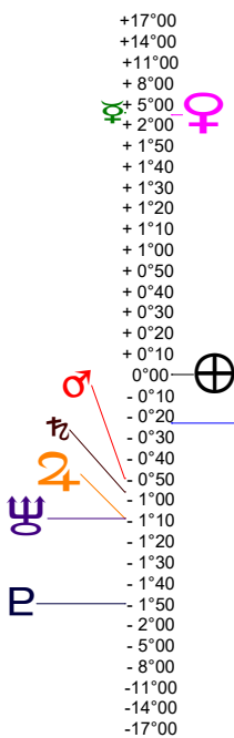
Latitudes héliocentriques
